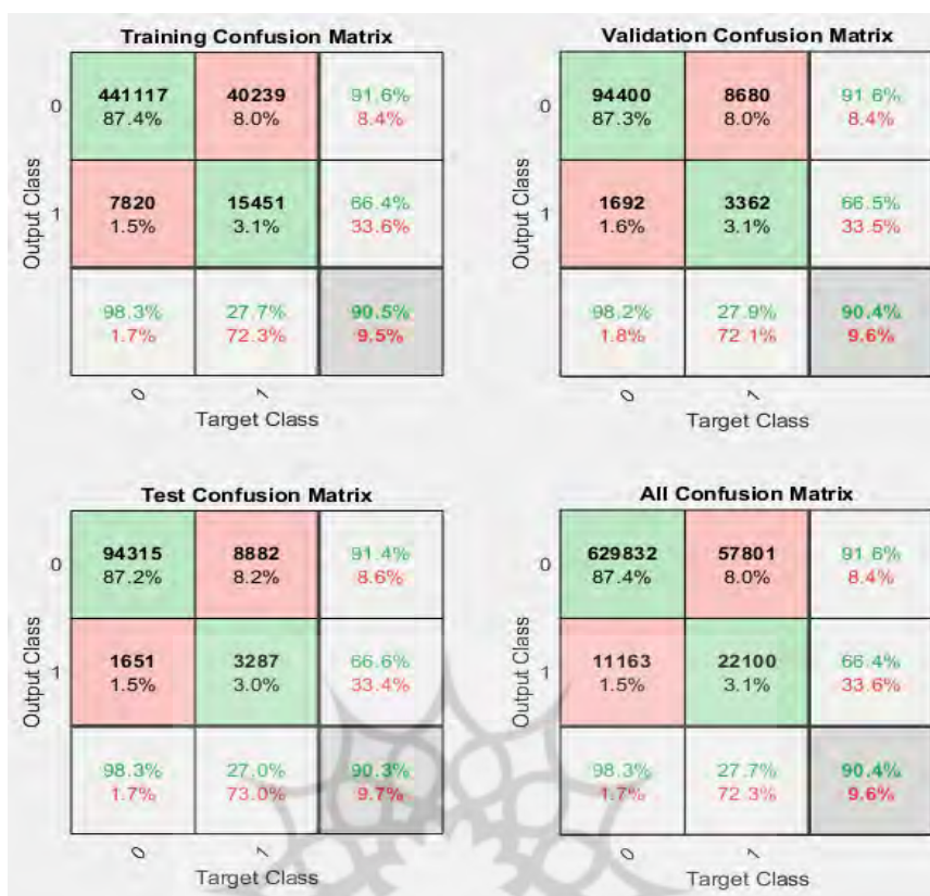
شکل ۱۸. نمودار دسته‌بندی و کارایی تخمین شبکه عصبی
