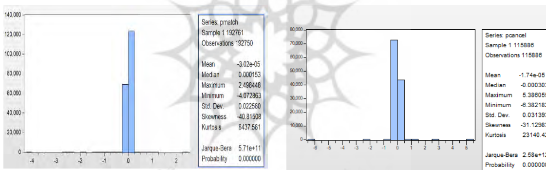
شکل ۷. نمودار پراکندگی و آزمون کشیدگی و چولگی شکل ۸. نمودار پراکندگی و آزمون کشیدگی و چولگی قیمت‌های کنسلی قیمت‌های تطبیق یافته
