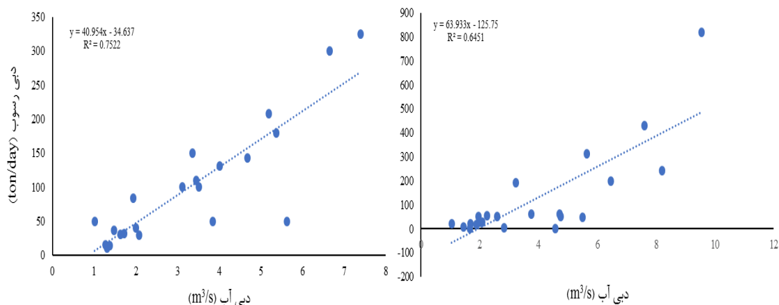
شکل ۱۱. منحنی سنج رسوب ایستگاه گلورد (فصل بهار)
