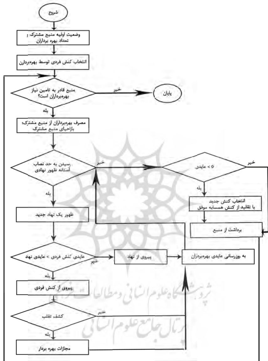
شکل ۲. فلوجارت فرآیند شبیه سازی مدل نهاد خودگردان
