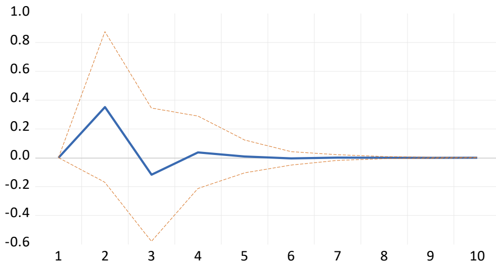
نمودار ۸: تابع واکنش آنی پاسخ بخش خدمات به شوک بخش معدن (منبع: یافته‌های پژوهش)
