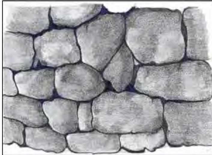
شکل ۱۰: طرحی از نحوه چیدمان خشکه‌چین بنای سنگی (طرح: نگارندگان، ۱۳۹۸).
