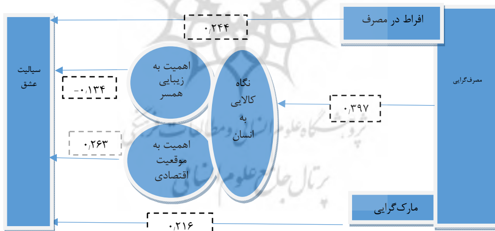
نمودار ۲. تحلیل مسیر
