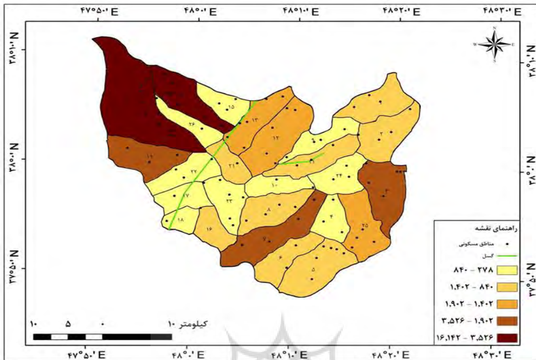
شکل ۵- نقشه پراکندگی مقادیر شاخص گرادیان طولی رود در منطقه مورد مطالعه
