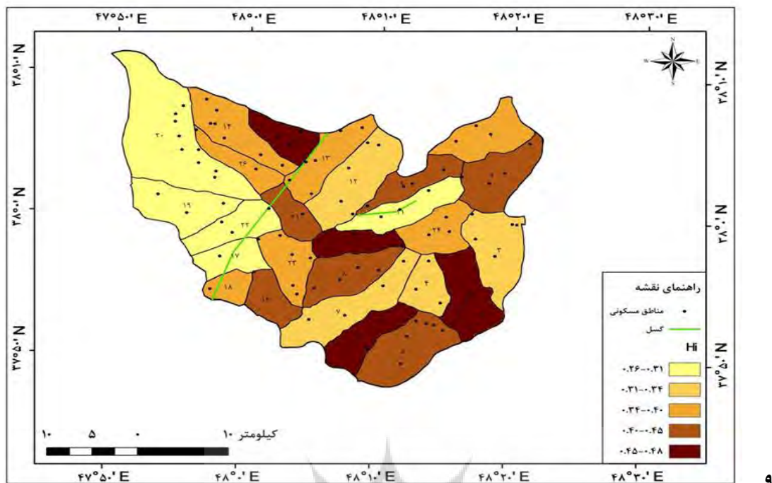
شکل ۶- نقشه پراکنندگی شاخص انگرال فراژسجی در منطقه مورد مطالعه
