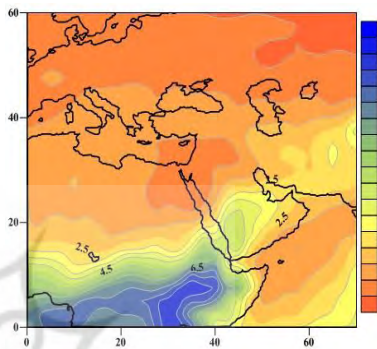
شکل ۲۰. نقشه متوسط رطوبت ویژه (به گرم در کیلوگرم) تراز ۷۰۰ هکتوپاسکال در زمان استقرار الگوی شماره ۵
