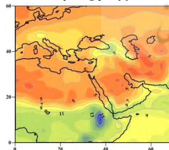
شکل ۸ - نقشه متوسط رطوبت ویژه (به گرم در کیلوگرم) تراز ۸۵۰ هکتوپاسکال در زمان استقرار الگوی شماره ۲
