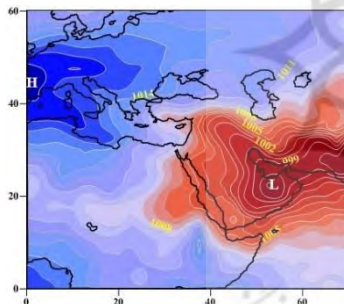
شکل ۵ - نقشه متوسط رطوبت ویژه (به گرم در کیلوگرم) و شکل ۶ - نقشه متوسط فشار تراز دریا (به میلی بار) در زمان تراز ۱۰۰۰ هکتوپاسکال در زمان استقرار الگوی شماره ۲
