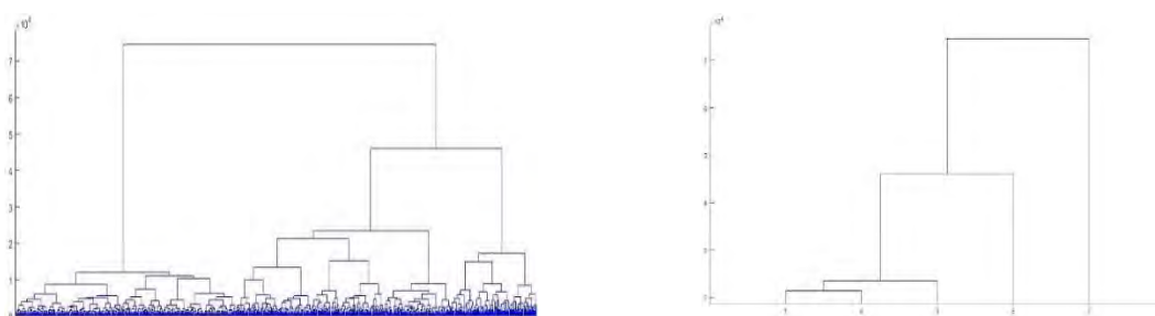
شکل ۲. نمودار درختی کل الگوهای گردشی ناهمواری ارتفاع ژئوپتانسیل تراز ۵۰۰ هکتوپاسکال و ۵ الگوی اصلی در طی دوره
