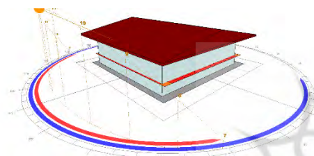
شکل ۴. نمونه طراحی شده در حالت اول طراحی فضای کاملاً شیشه‌ای بدون پوسته
