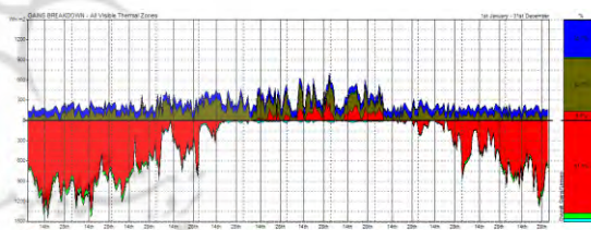
شکل ۲۱. نمودار شکست دریافت/ اتلاف حرارت ( Passive Gain Breakdown) - برای حالت سوم
