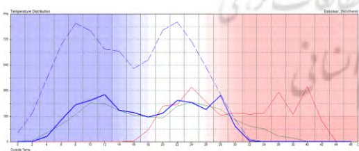
شکل ۱۶. نمودار توزیع دمایی (Temperature Distribution) - برای حالت سوم
