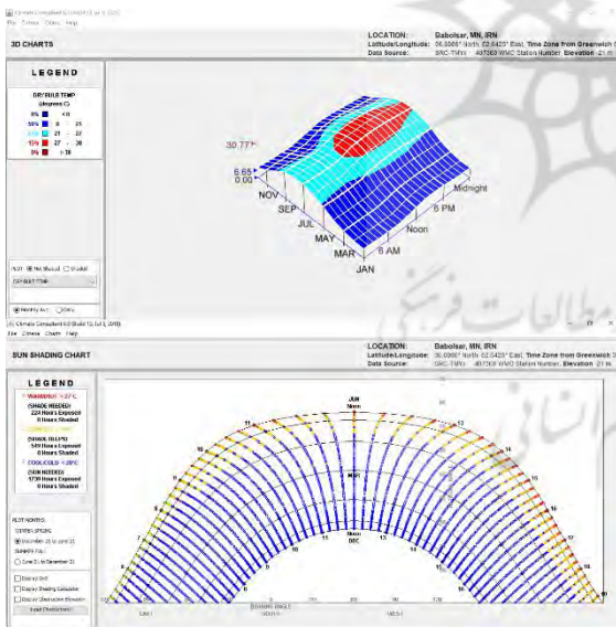
شکل ۱۰. نمودار تحلیل و بررسی زاویه تابش خورشید برای سایه‌اندازی در شهرستان بابلستر - مأخذ: (نرم‌افزار مشاور انرژی)
