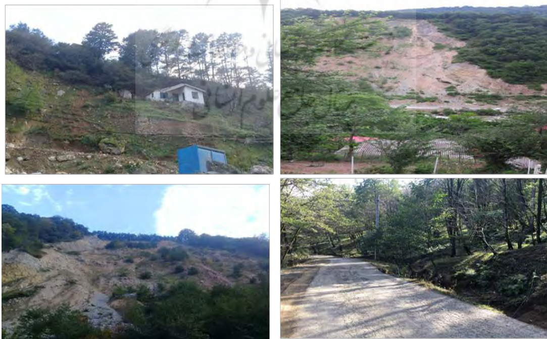
شکل ۱۵. تصاویری از نقش عوامل طبیعی و انسانی در وقوع زمین لغزش در حوضه آبخیز خانیان
