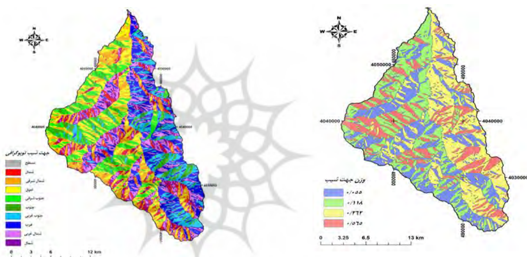
شکل ۹. نقشه جهت شیب و وزندهی جهت چهارگانه
