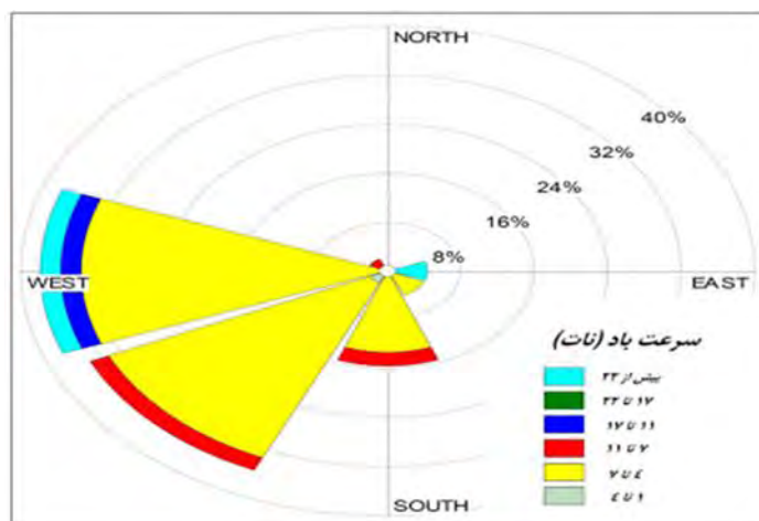
شکل ۸. گلباد ایستگاه هواشناسی تنکابن
