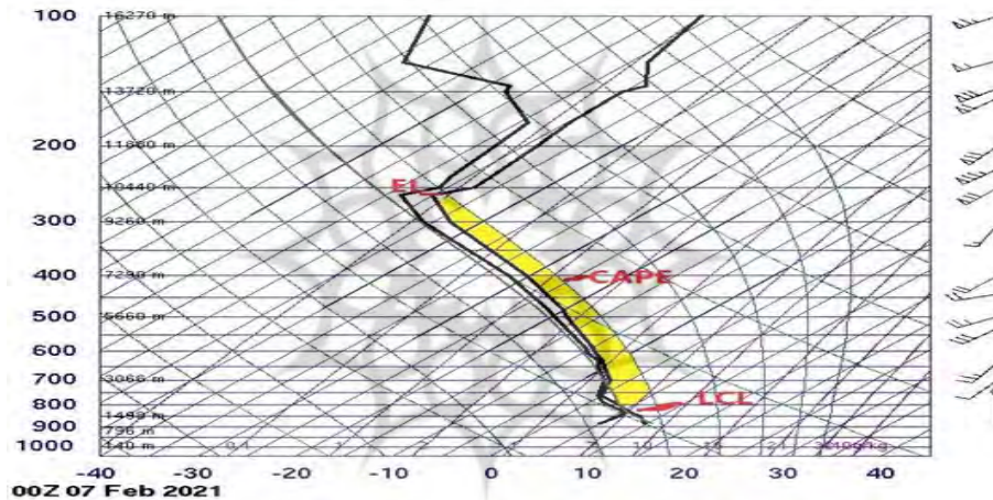
شکل ۸. نمودار اسکیتوتی برای سناریو دوم، جو ناپایدار شاخص آلودگی ناسالم
