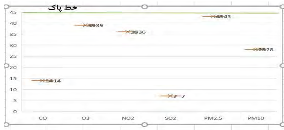
شکل ۱۳. میانگین انتشار روزانه آلاینده‌ها در ۵ ایستگاه محدوده مطالعه در سناریو سوم
