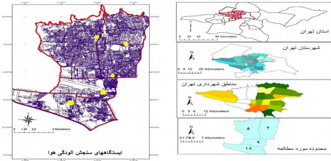
شکل ۱. نقشه محدوده مورد مطالعه (سمت راست) و موقعیت ایستگاه‌های اندازه‌گیری آلودگی هوا (سمت چپ)
