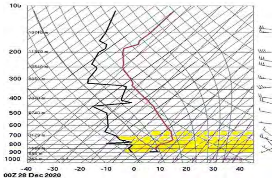
شکل ۵. نمودار اسکویته برای روز ۲۸ دسامبر ۲۰۲۰، روز ناسالم از لحاظ شدت آلودگی
