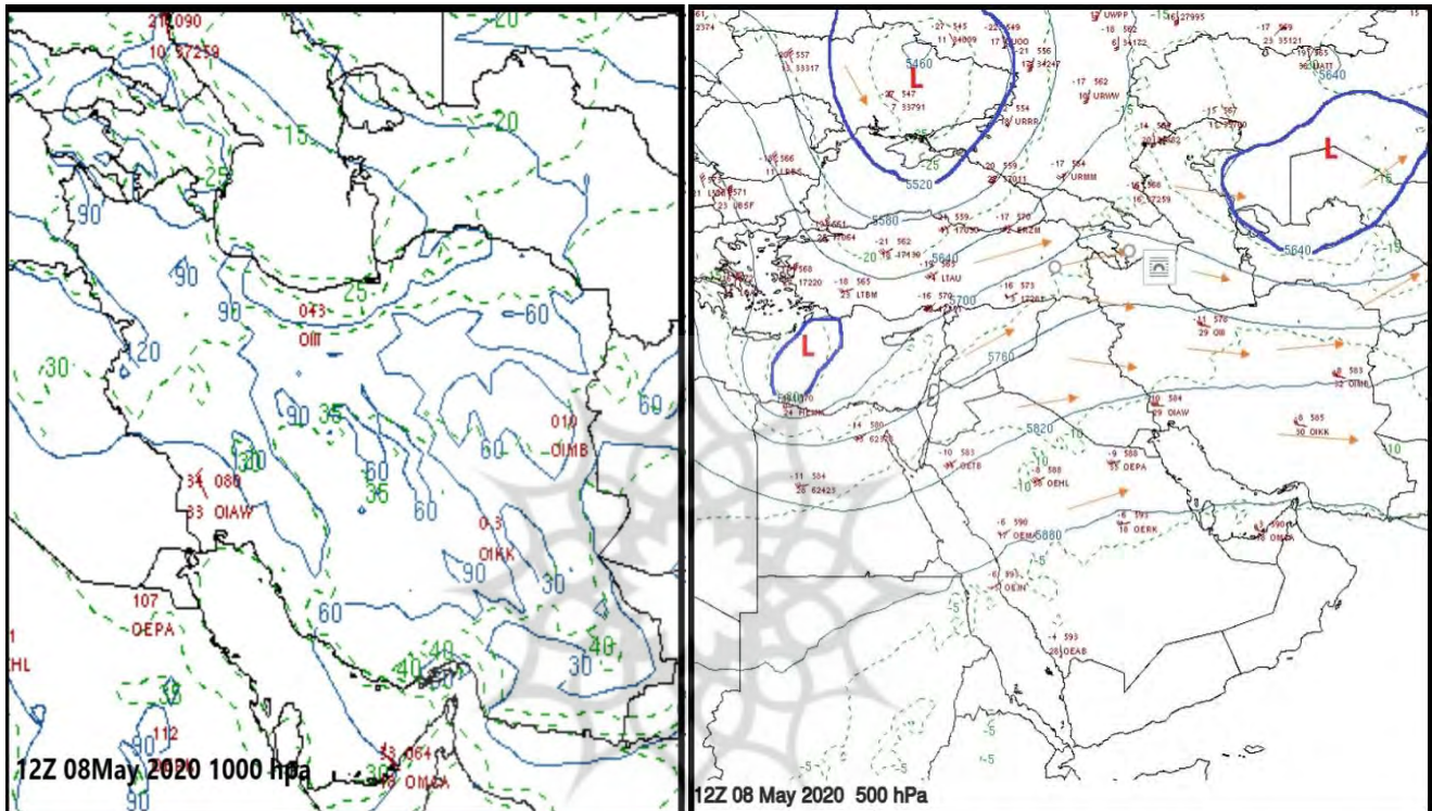
شکل ۱۲. نقشه‌های تراز ۱۰۰۰ و ۵۰۰ هکتوپاسکال بر اساس الگوی سناریوی سوم
