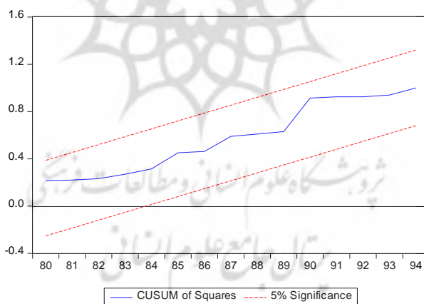
نمودار ۲. آزمون گرافیکی CUSUMQ.
