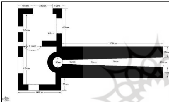
ت ۵. پلان آسیاب آبی شیخ مکان ۱ با استناد به بقای معماری برجای مانده از آن (منبع: نگارنده).
