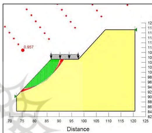
ن 1. بحرانی‌ترین سطح لغزش شیروانی خاکی در حالت خشک با استفاده از نرم‌افزار Geoslope-7.10.
