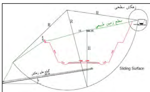
ن 3. مکانیزم زمین لغزش و طرح پایدارسازی مربوط به آن (H عمق لغزش و R شعاع لغزش).
