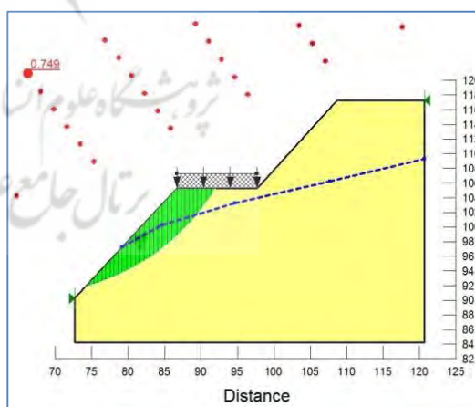
ن 2. بحرانی‌ترین سطح لغزش در توده لغزنده در حالت اشباع با استفاده از نرم‌افزار Geoslope-7.10.
