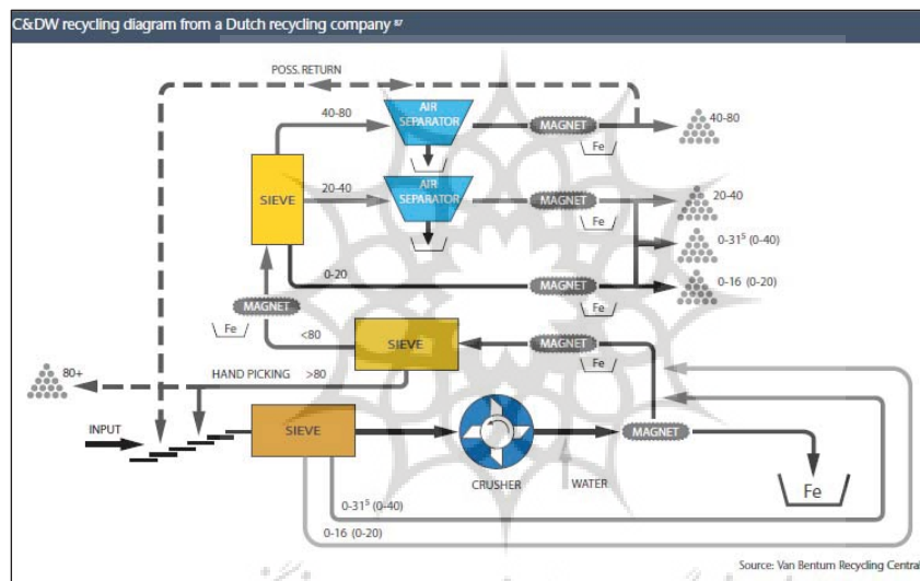
ت ۴. تصویر شماتیک از فرایند بازیافت بتن.
