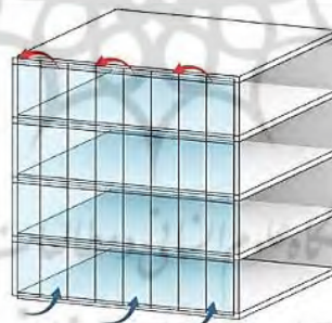
تصویر ۹: نما دو پوسته چند طبقه (Ajla Aksamija, ۲۰۱۸)
