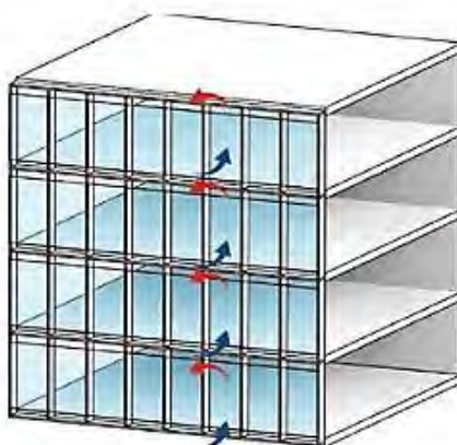
تصویر ۱۳: نما دوپوسته پنجره ای جعبه ای (Ajla Aksamija, ۲۰۱۸)
