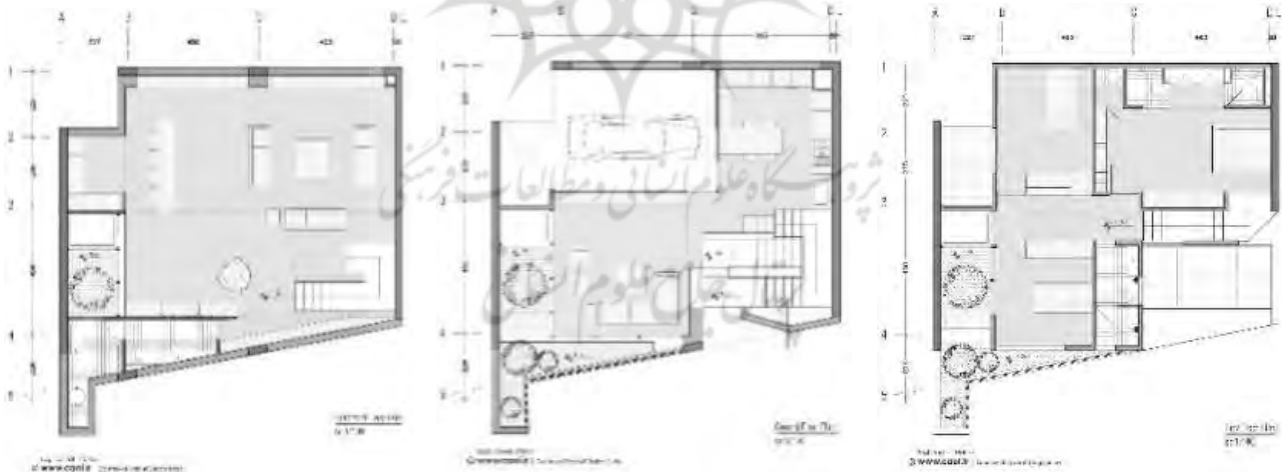
تصویر ۱۱. پلان‌های معماری خانه جنت. مأخذ: www.caoi.ir
