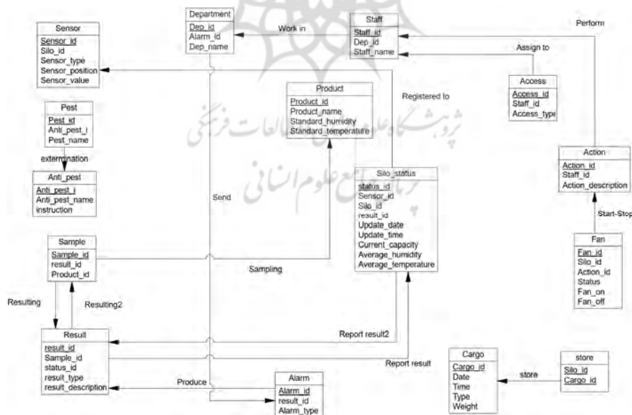
شکل ۳. مدل فیزیکی به کارگیری اینترنت اشیا در بخش ذخیره‌سازی زنجیره تأمین گندم
