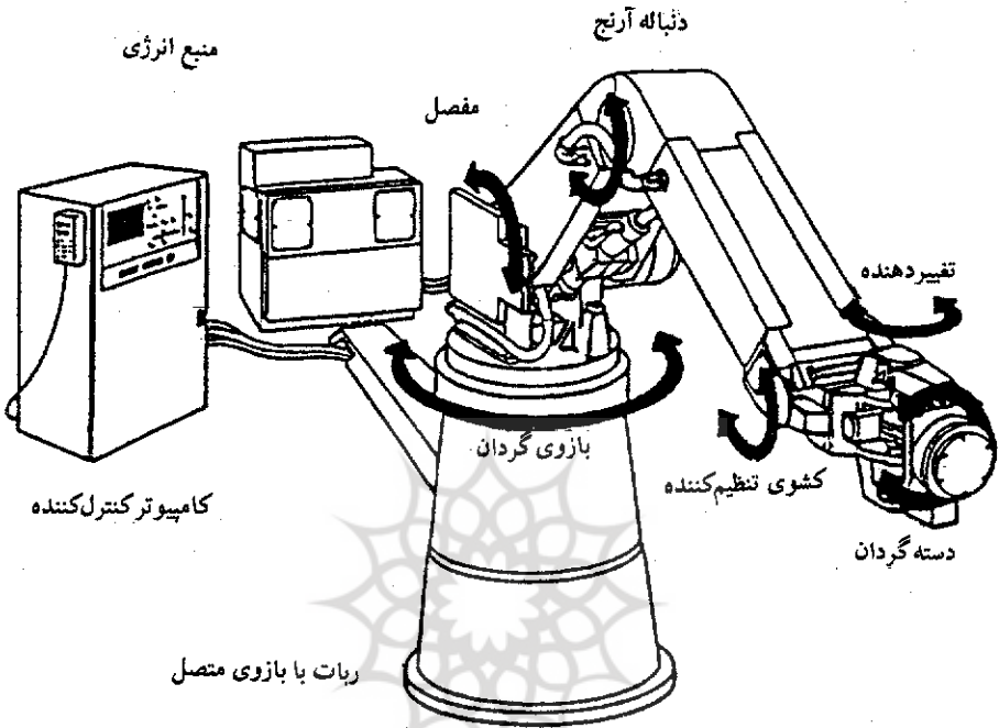
شکل (۱) - اجزای تشکیل دهنده ربات
