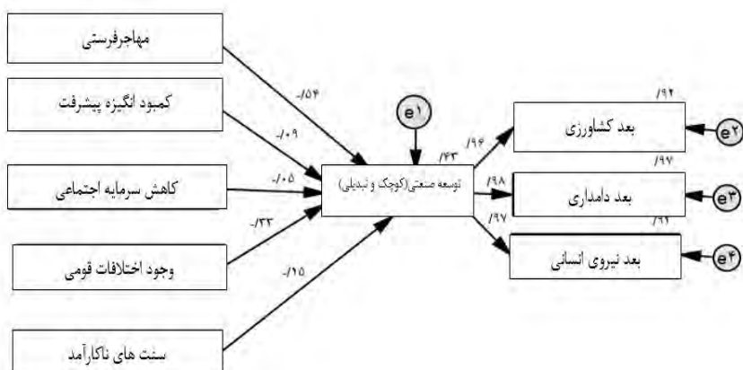
شکل شماره ۳: وزن های رگرسیونی استاندارد شده
