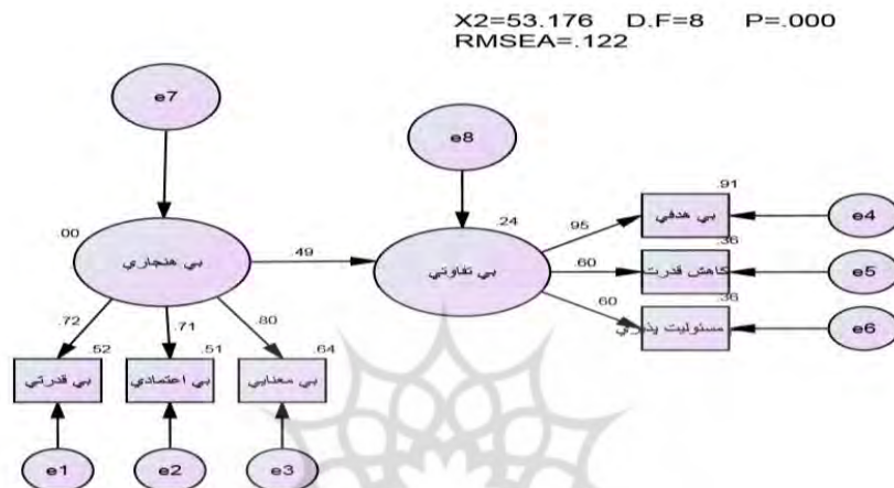
نمودار(۲) مدل برازش شده در حالت ضرایب استاندارد شده
