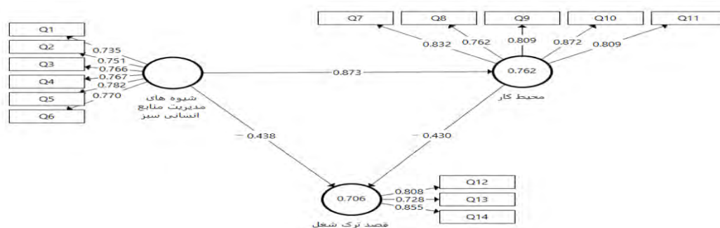
شکل ۲- ضرایب مسیر
