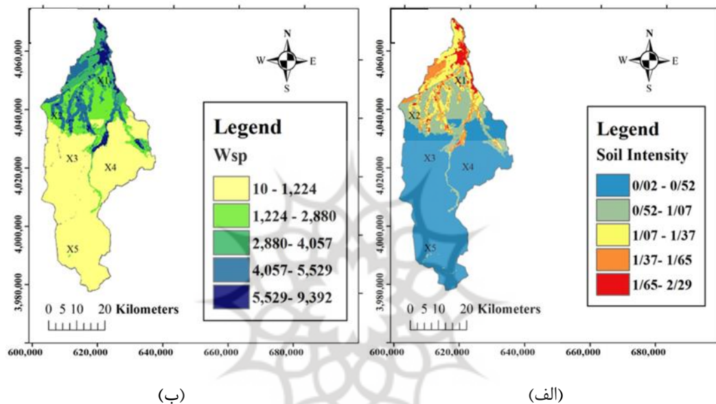
شکل (۳). (الف) ضریب شدت فرسایش در حوزه آبریز بابلرود، (ب) میانگین سالانه فرسایش ویژه در حوزه آبریز بابلرود
