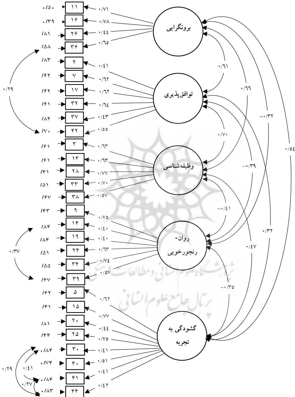
شکل ۱. نمودار مدل نهایی همراه بارهای عاملی کاملاً استاندارد شده
