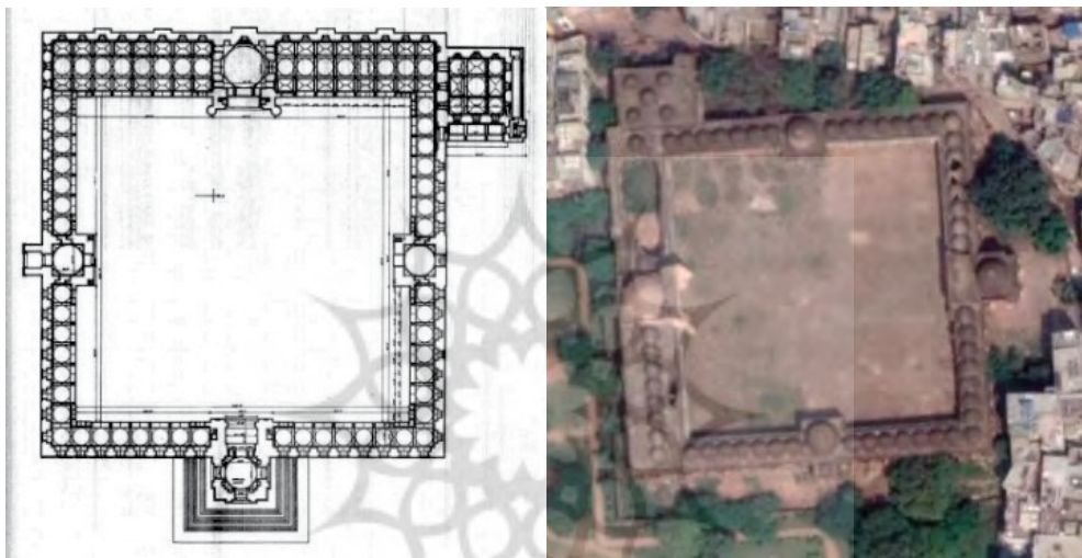
تصویر ۱۱- پلان مسجد جهان‌پناه. مأخذ: (Welch, 1983, 131) و تصویر هوایی آن. مأخذ: (URL 8)
