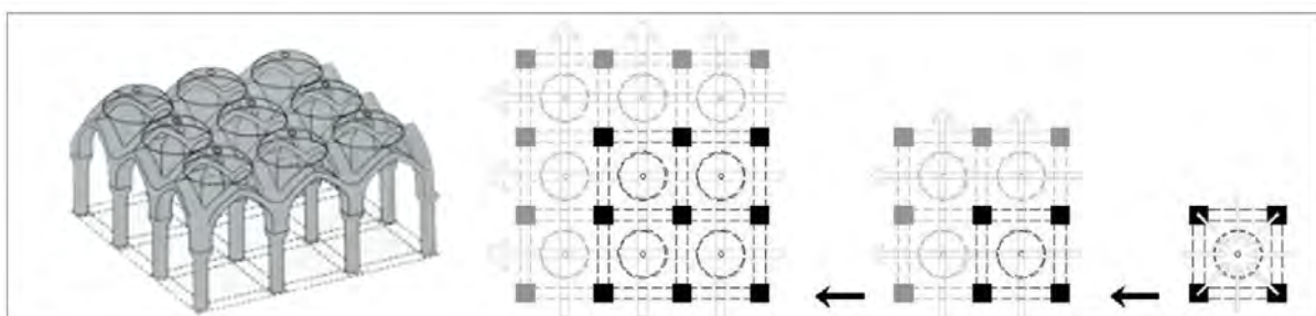
تصویر ۱- راست: شکل‌گیری شبستان نه‌گنبد از تکرار چهارطاقی. چپ: نمود فرمی شبستان نه‌گنبدی. مأخذ: (نویایی و حاجی قاسمی، ۱۳۹۰).
