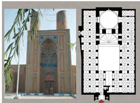
تصویر ۱۹- اولین نمودهای دستگاه ورودی، جامع اشترجان ایلخانی. ماخذ: (گنجنامه، مساجد جامع)
