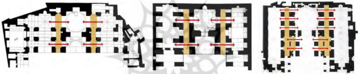
تصویر ۲۳- پیوستگی ساختاری گنبدخانه و شبستان با شکل‌گیری مفصل فضایی، راست: جامع یزد (ایلخانی)، وسط: جامع ورزنه (تیموری)، چپ: مسجد حکیم (صفوی).
