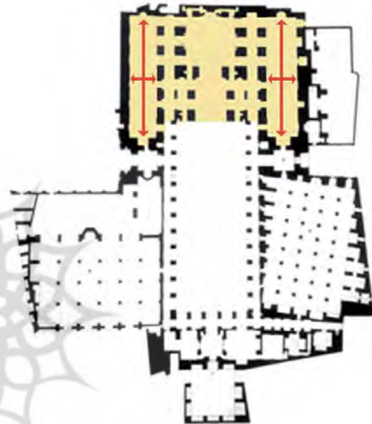
تصویر ۱۲- افزایش پیوستگی بصری شبستان با افزایش عرض دهانه‌ها، مسجد جامع یزد، صفوی. (مرکز اسناد سازمان میراث فرهنگی اصفهان)
