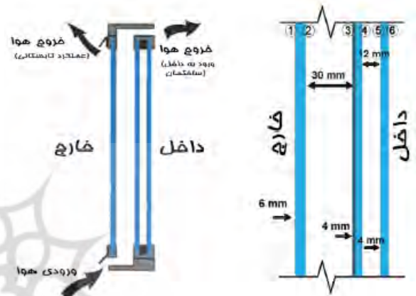
تصویر- سمت چپ: شکل شماتیک پنجره ی دمنده ی هوا و سمت راست: پیکربندی شماره ۲ با پوشش لایه ی کم گسیل روی سطح ۳ (از خارج).
