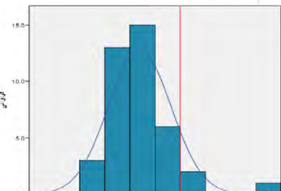
نمودار چگونگی توزیع میزان تاب‌آوری شهر تبریز در بعد مدیریتی
