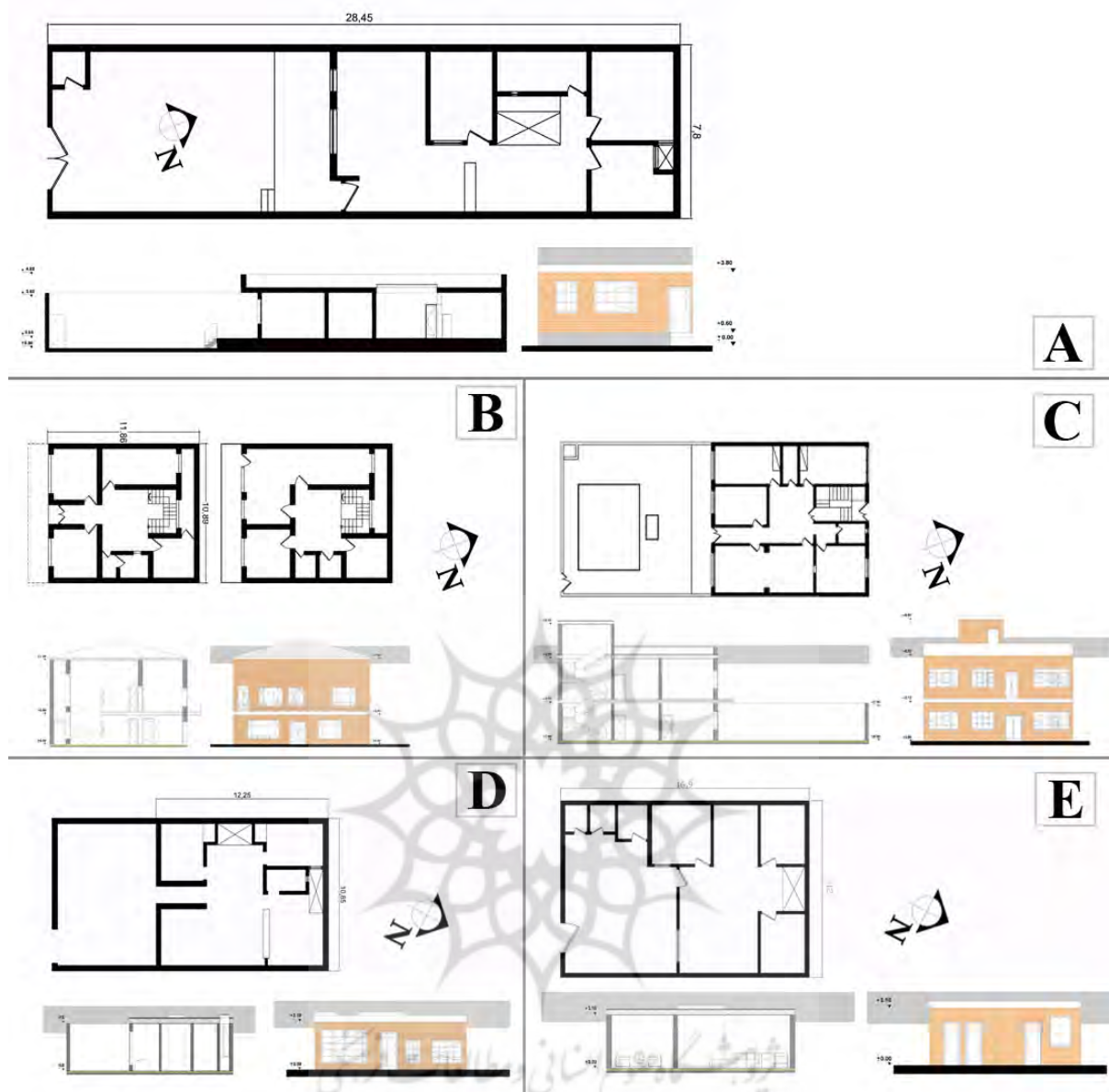
تصویر ۱- پلان، نما و مقطع تعدادی از نمونه‌های موردی؛ A: خانه شماره ۳ یک طبقه با هم‌جواری هم‌پلاک از گروه ۱؛ B: خانه شماره ۱ دوطبقه با هم‌جواری هم‌پلاک از گروه ۱؛ C: خانه شماره ۷ دو طبقه با هم‌جواری هم‌پلاک از گروه ۱؛ D: خانه شماره ۴ یک طبقه با هم‌جواری هم‌پلاک از گروه ۲؛ E: خانه شماره ۶ یک طبقه با هم‌جواری هم‌پلاک از گروه ۲.
