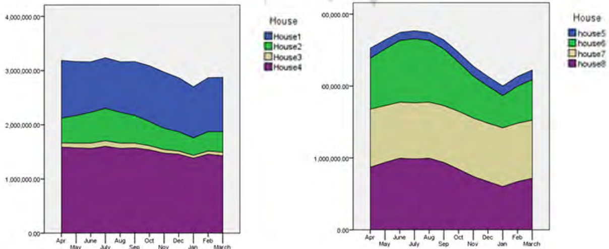
تصویر ۳- انرژی تابیده شده بر بدنه‌های خانه‌های گروه ۱ و ۲.
