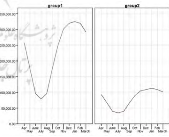
تصویر ۱۲- میانگین انرژی خورشیدی تابیده شده بر بدنه‌های عمودی ساختمان در گروه ۱ و ۲.
