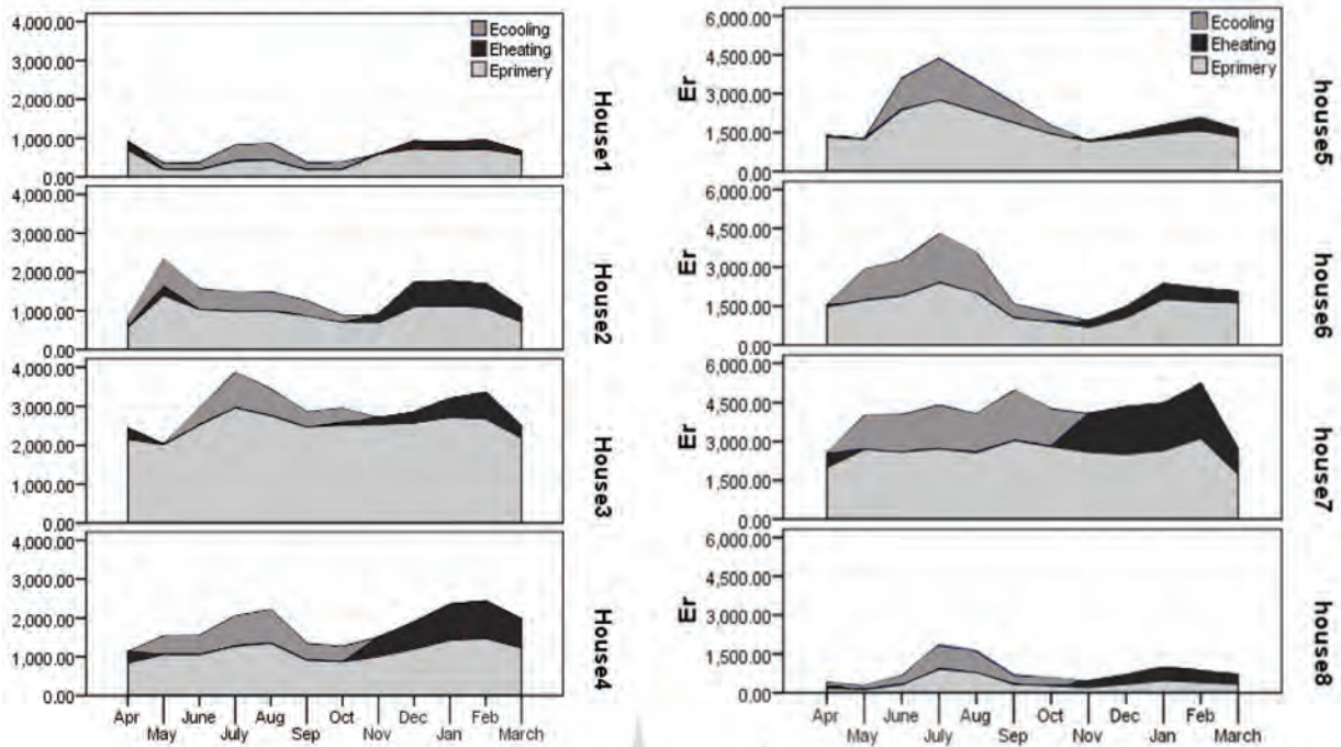
تصویر ۲- مصرف انرژی اولیه، سرمایش و گرمایش در گروه ۱ و ۲.
