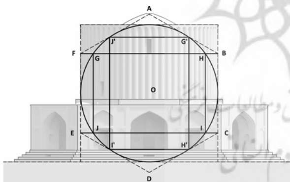
تصویر ۱۶ - ترسیم مستطیل \frac{1}{2}\sqrt{2} و یافتن سطح همکف.
