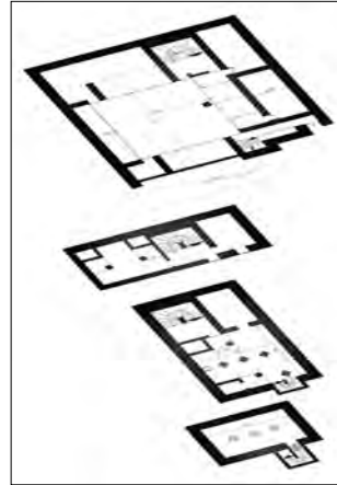
تصویر ۲۱ و ۲۲- پلان همکف، سرداب اول، دوم و سوم و تصویری از ایوان اصلی داخلی خانه ابومشتاق؛ تراس کوچک کار شده در نیم طبقه ایوان نشان از تلاش معمار در استفاده از لایه‌های مختلف ارتفاعی در خانه دارد.
