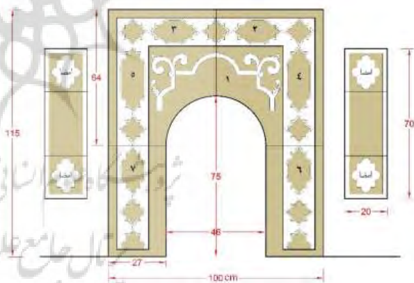
تصویر ۱- قاب بندی شومینه موزه اولانا.
