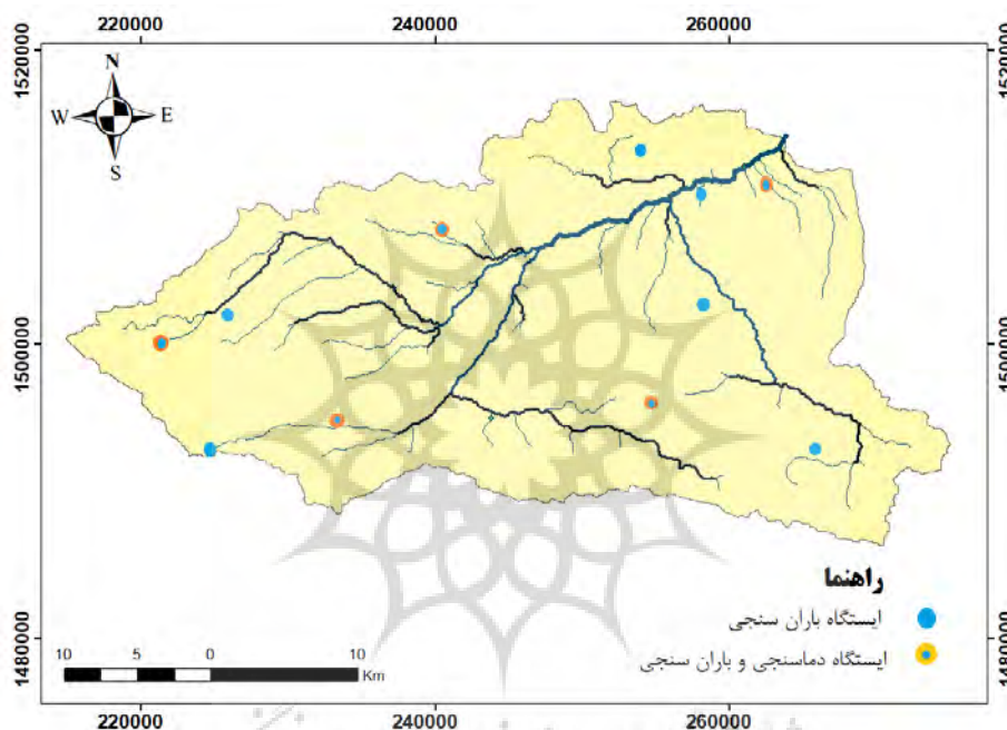
شکل ۳- موقعیت ایستگاه‌های هواشناسی و شبکه آبراهه‌ای آبخیز سملقان.
