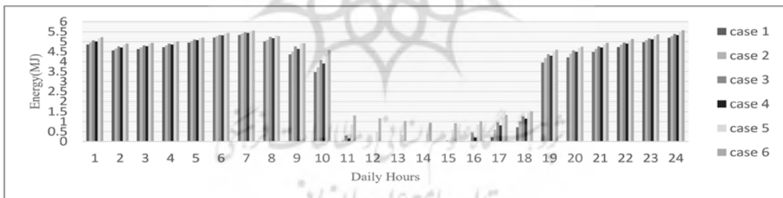
نمودار ۲- میزان مصرف انرژی سرمایه‌ش در روز- طرح زمستان.
