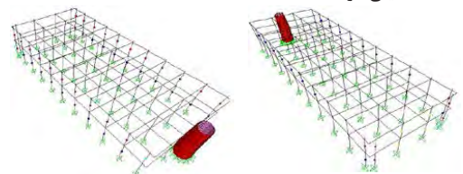
تصویر ۱۶- وضعیت مفاصل پلاستیک تشکیل شده در سازه تحت الگوی بار جانبی مثلثی تحت بار ثقلی 1.1(dead+0.25live) برای قسمت یک طبقه الف) در راستای طولی ساختمان در تغییر مکان هدف ۱۱ میلی‌متر، ب) در راستای عرضی ساختمان در تغییر مکان هدف ۵۱ میلی‌متر.
