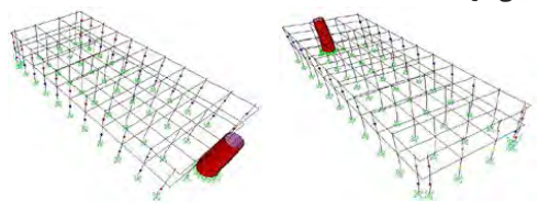
تصویر ۱۵- وضعیت مفاصل پلاستیک تشکیل شده در سازه تحت الگوی بار جانبی مثلثی تحت بار ثقلی 0.9dead برای قسمت یک طبقه الف) در راستای طولی ساختمان در تغییر مکان هدف ۱۱ میلی‌متر، ب) در راستای عرضی ساختمان در تغییر مکان هدف ۵۱ میلی‌متر.
