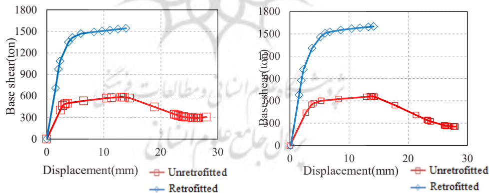
تصویر ۲۰- مقایسه منحنی‌های پوش‌آور ساختمان مورد مطالعه قبل و بعد از مقاوم‌سازی تحت الگوی بار ثقیلی 0.9dead و الگوی بار جانبی مثلثی، الف) در راستای طولی، ب) در راستای عرضی.
