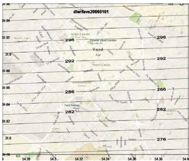
شکل (۹) شار ورودی موج بلند ساعت ۹ (منبع CFSR)
