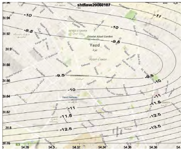
شکل (۱۹) شار گرمای محسوس ساعت ۷ (منبع CFSR)
