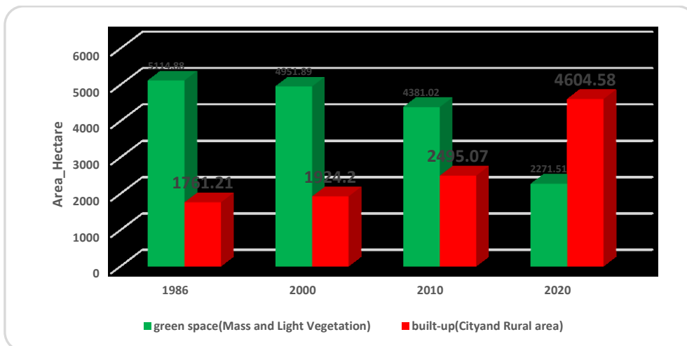
نمودار ۵: تغییرات کاربرد زمین در شهر آمل برای سال 1986, 2000, 2010 و ۲۰۲۰
