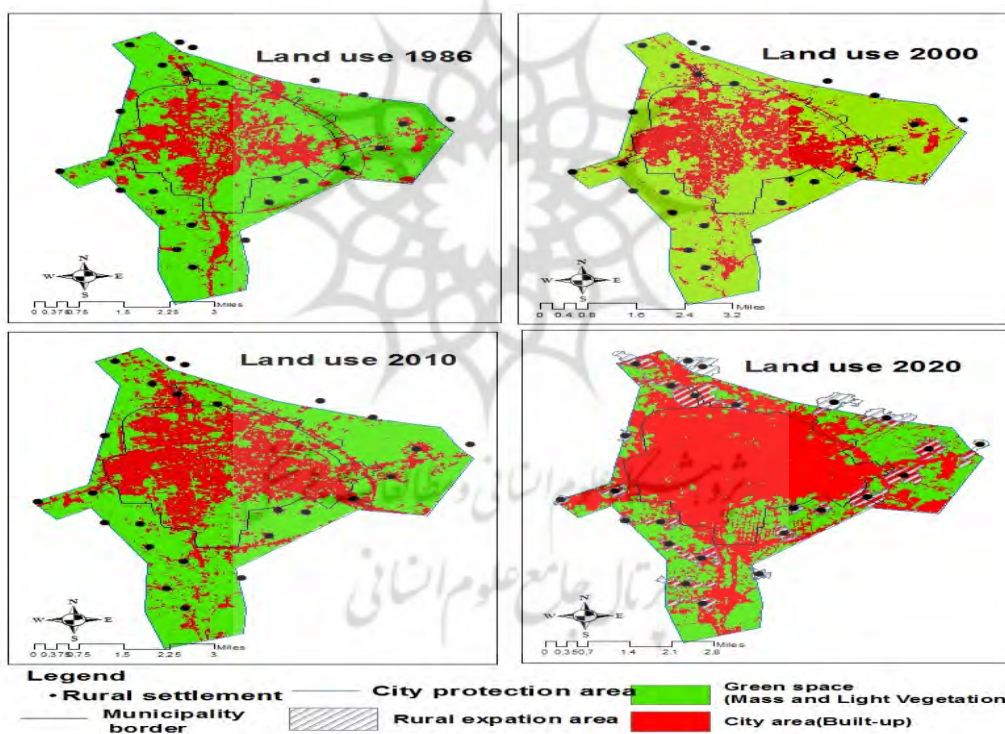
شکل ۳: روند رشد شهری در سال‌های ۱۹۸۶, 2000, 2010 و ۲۰۲۰
