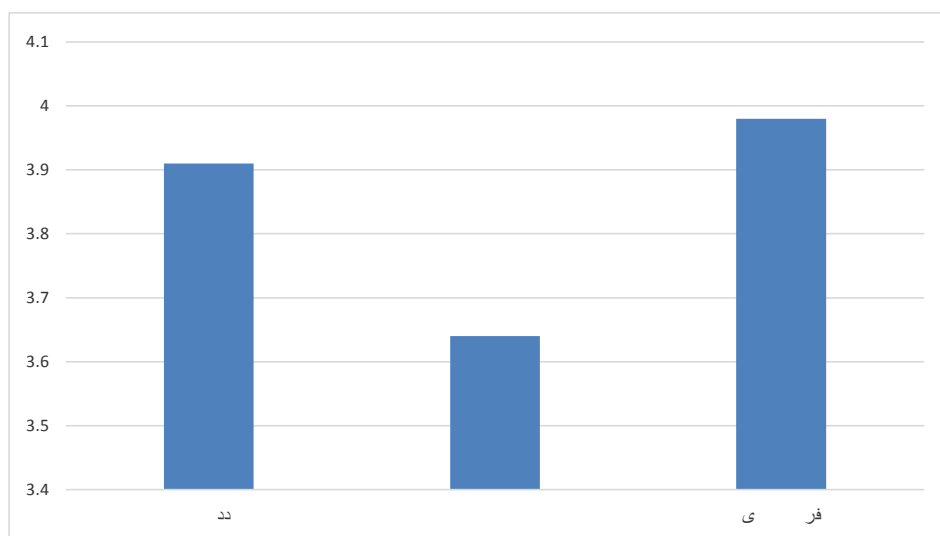
نمودار ۱. آمار توصیفی مهمترین موانع همگرایی روابط ایران و مصر، منبع: (ترسیم نگارندگان)
