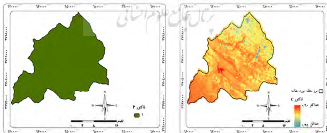
شکل ۸: نقشه عملیات حفاظتی فاکتور (P)
