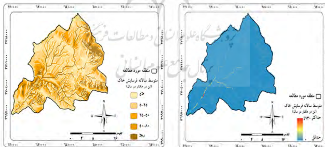
شکل ۱۰: نقشه کلاس خاک
