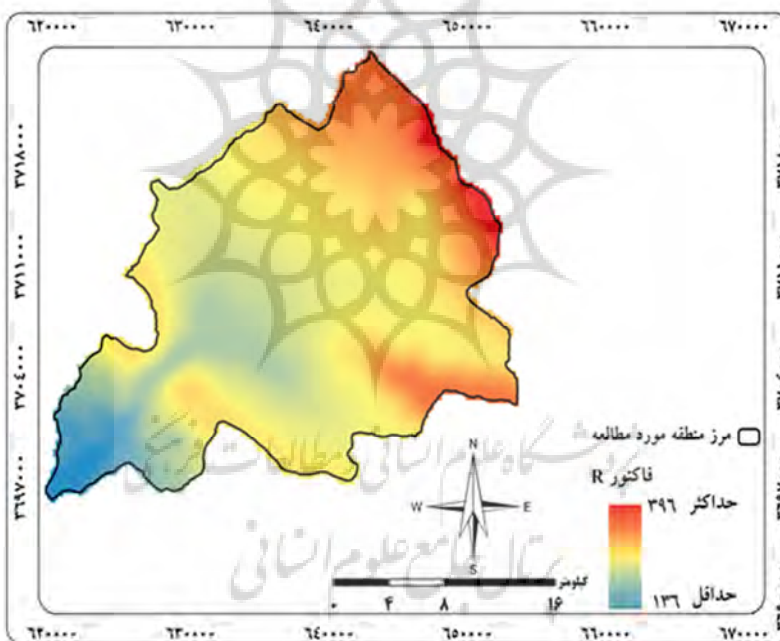
شکل ۴: نقشه عامل فاکتور R
