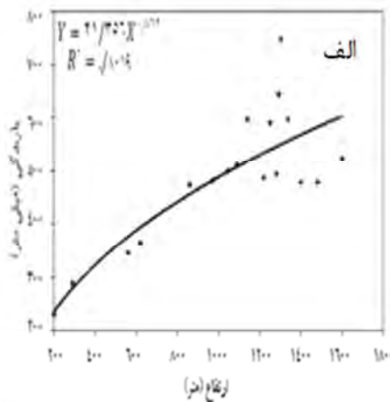
شکل ۲: رابطه بین ارتفاع و بارندگی
