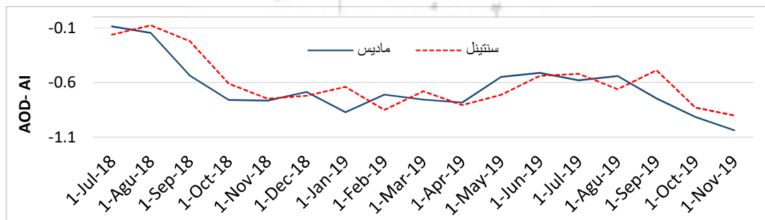
شکل ۳: روند تغییرات میانگین ماهانه آئروسول در محدوده مطالعاتی در ۲ سال اخیر (منبع: نگارندگان)
