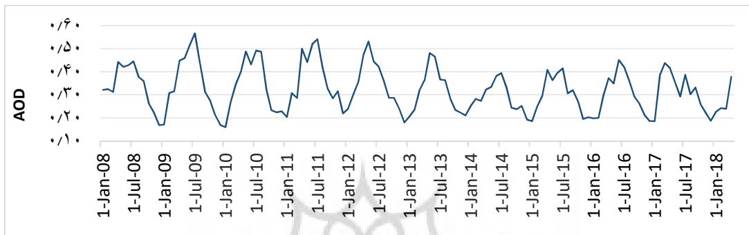
شکل ۲: روند تغییرات میانگین ماهانه در محدوده مطالعاتی در ۱۰ سال اخیر (منبع: نگارندگان)
