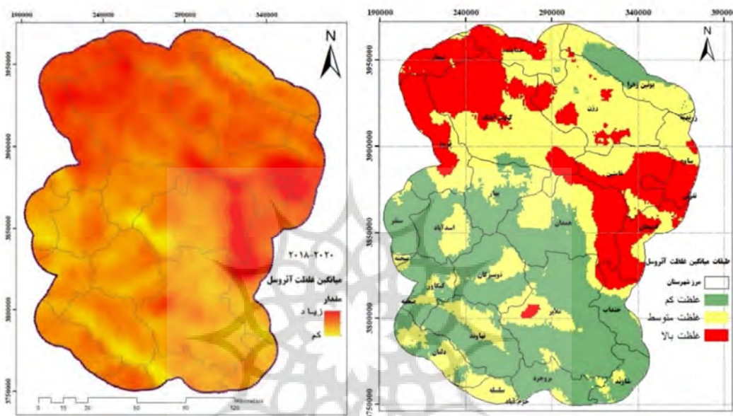
شکل ۶: میانگین ماهانه غلظت آتروسل (سمت چپ) و طبقه‌بندی آن (سمت راست) در سال ۲۰۱۸-۲۰۲۰ (سنتینل) (منبع: نگارندگان)
