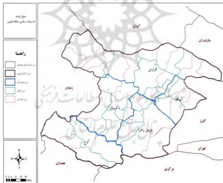
شکل ۶. منطقه‌بندی اداری-سیاسی
