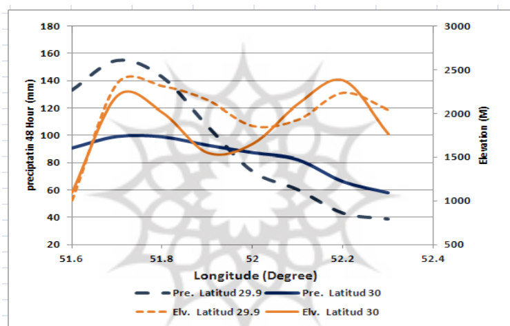
شکل (۱۰). تغییرات بارش با ارتفاع و طول جغرافیایی در عرض جغرافیایی ۲۹/۹ و ۳۰ درجه توفان مورخ ۱۴ تا ۱۵ آذر ۱۳۸۲ در محدوده حوضه سد پارسین
