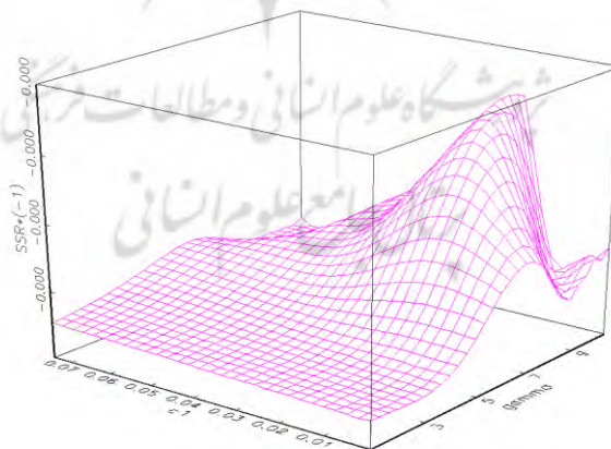
شکل ۱. قرینه تابع مجموع مربعات خطا
