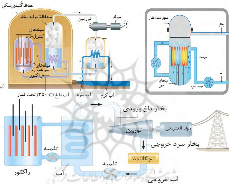
تصویر ۱۰. بخش‌ها و عملیات صورت گرفته در رآکتورهای هسته‌ای؛ ماخذ: آرشيو نگارندگان.
