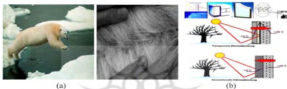
شکل ۱۱. ساختار TIW (الف) خرس قطبی با پوست سیاه و موی روشن؛ (ب) اصول عایق گرمایی TIW
