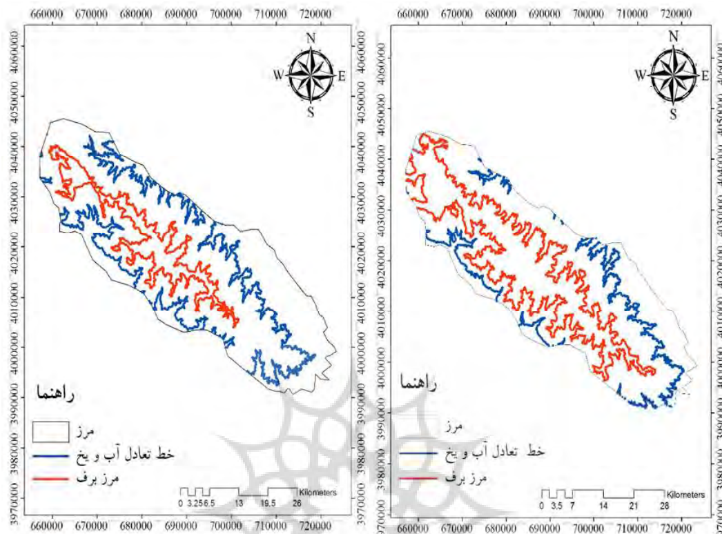
شکل شماره ۶. مرز برف دائمی و خط تعادل آب و یخ به روش نسبت‌های ارتفاعی؛ شکل شماره ۷. مرز برف دائمی و خط تعادل آب و یخ به روش نسبت مساحت تجمع
