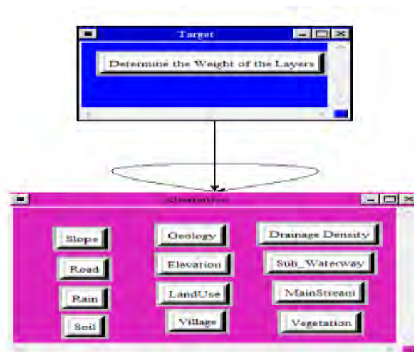
شکل ۲- ساختار تعیین ضریب اهمیت معیارها در نرم افزار Super Decision (یافته‌های پژوهش، ۱۴۰۰)
