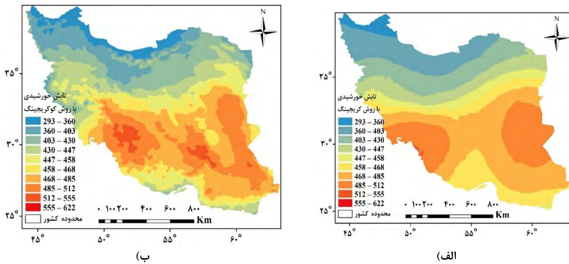
شکل ۶: خروجی پهنه‌بندی با روش کریجینگ عادی (OK): الف) بدون استفاده از داده کمکی
