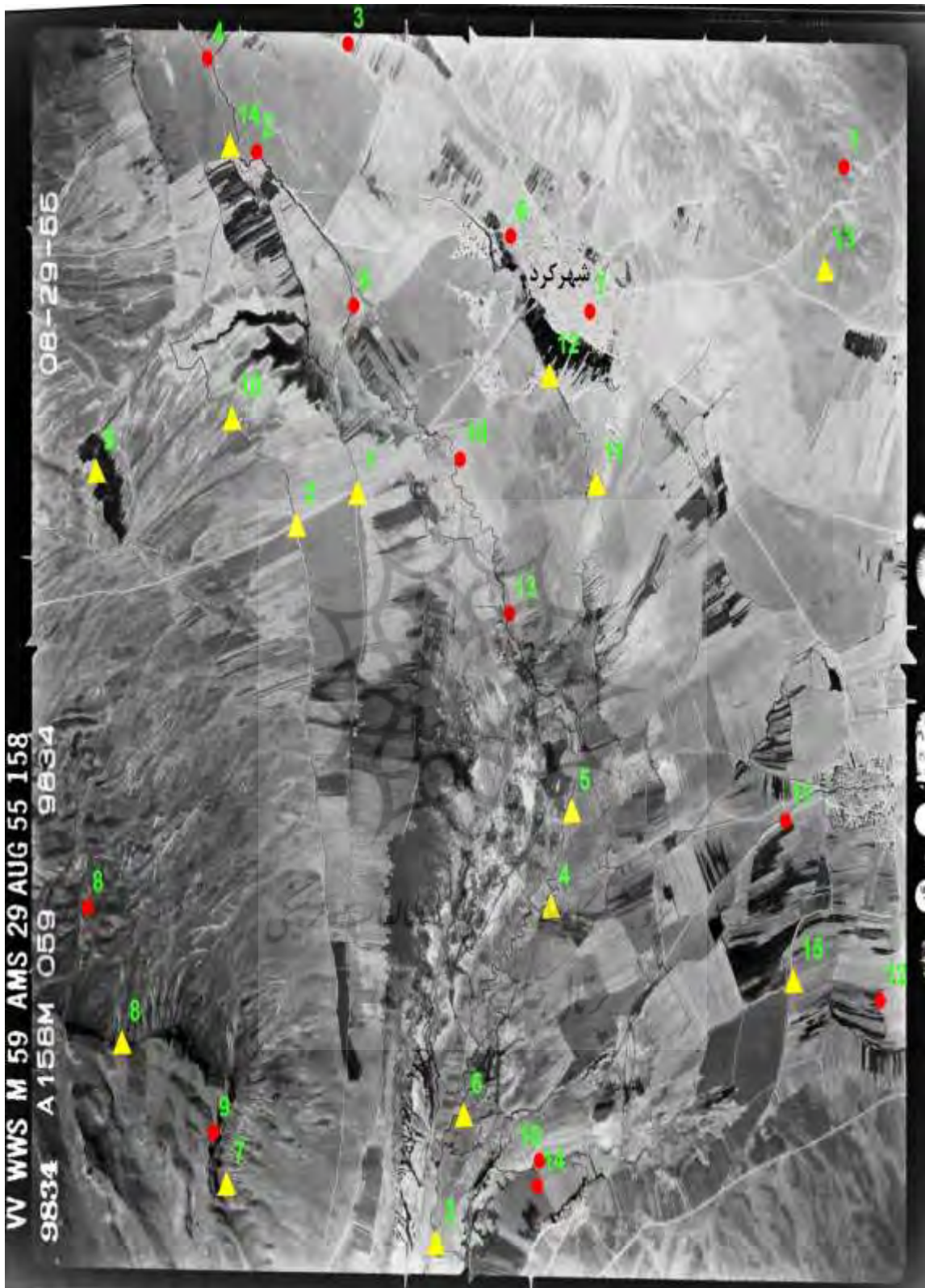
شکل (۳) عکس هوایی خام دشت شهرکرد به همراه نقاط شاهد زمینی (مثلث) و نقاط اندازه‌گیری خطا (دایره) Figure (3) Original aerial photograph of Shahrekord area with ground control points (triangle) and error measurement points (circle)
